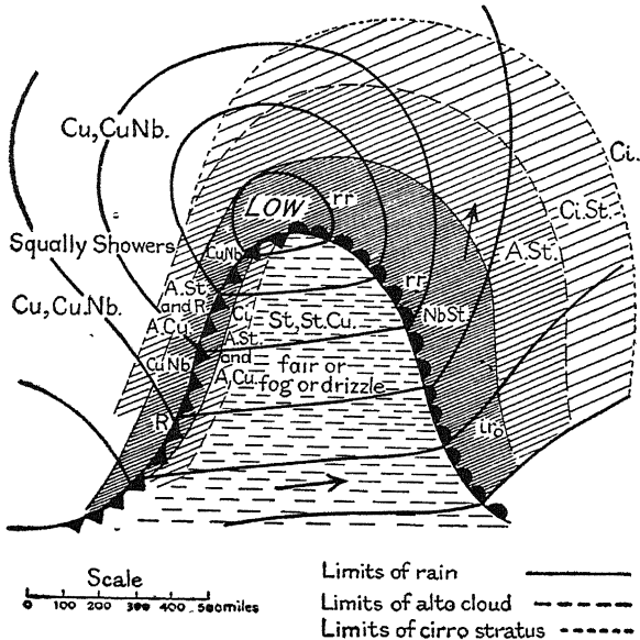
चित्र ५१ (a) — उष्णखंड में चक्रवात में बादल और मौसम
